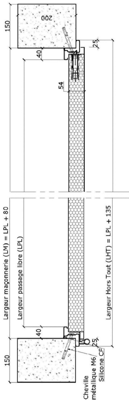
COUPE B-B ECH1:5
